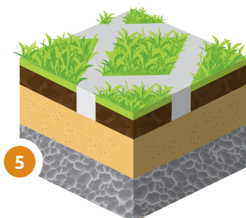
5 Dalles alvéolées
