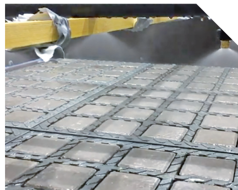
Test de perméabilité avec pluie artificielle sur dalles alvéolées et pavés bétons (© O2D)
